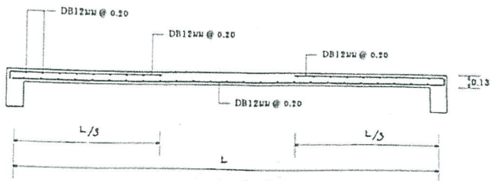
S16 รูปตัดด้านหนึ่ง
