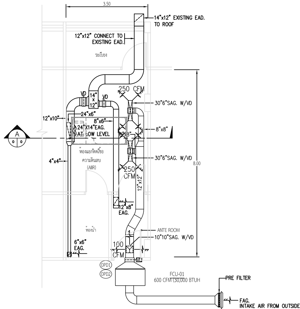
แบบระบบปรับอากาศ และระบายอากาศ
