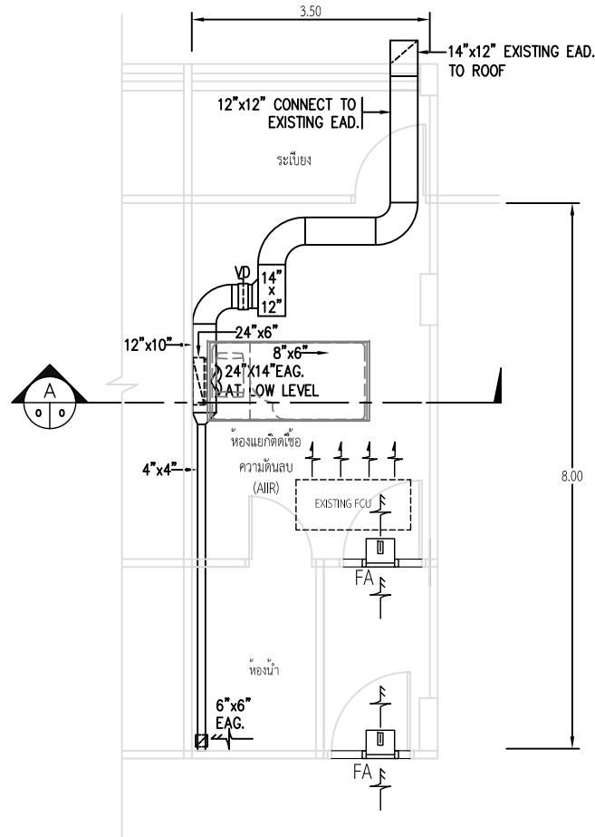
แบบระบบปรับอากาศ และระบายอากาศ
